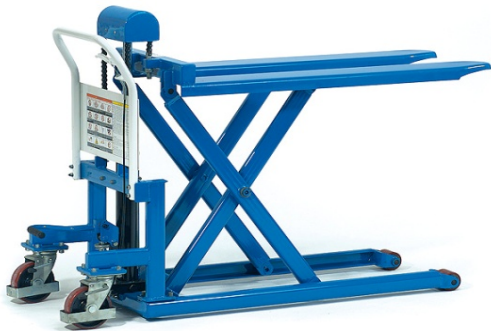
Scheren-Hubwagen 6820 - 500 kg
